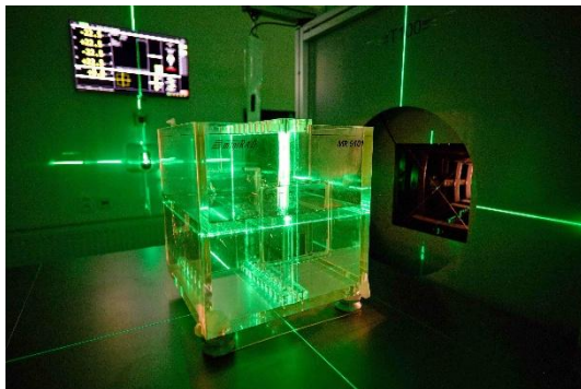
Zaměřování ozařování předmětu pomocnými lasery Foto: ÚJP PRAHA a.s. – Daniel Kasal
