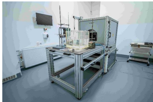
T100 se zapnutými zaměřovacími lasery Foto: ÚJP PRAHA a.s. – Daniel Kasal
