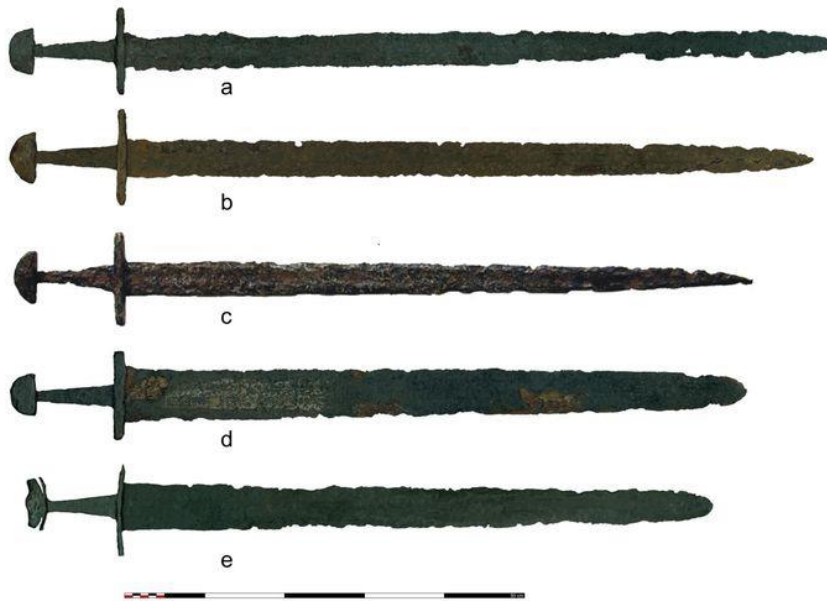
Tvarová rozmanitost čepelí mečů ze druhé poloviny 9. a raného 10. století nalezených na Moravě: a – Mikulčice-Valy, hrob 375; b – Nechvalín, grave 125; c – Mikulčice-Valy, hrob 438; d – Břeclav-Pohansko, hrob 26; e – Vranovice. FOTO: J. Hošek a J. Košta.
