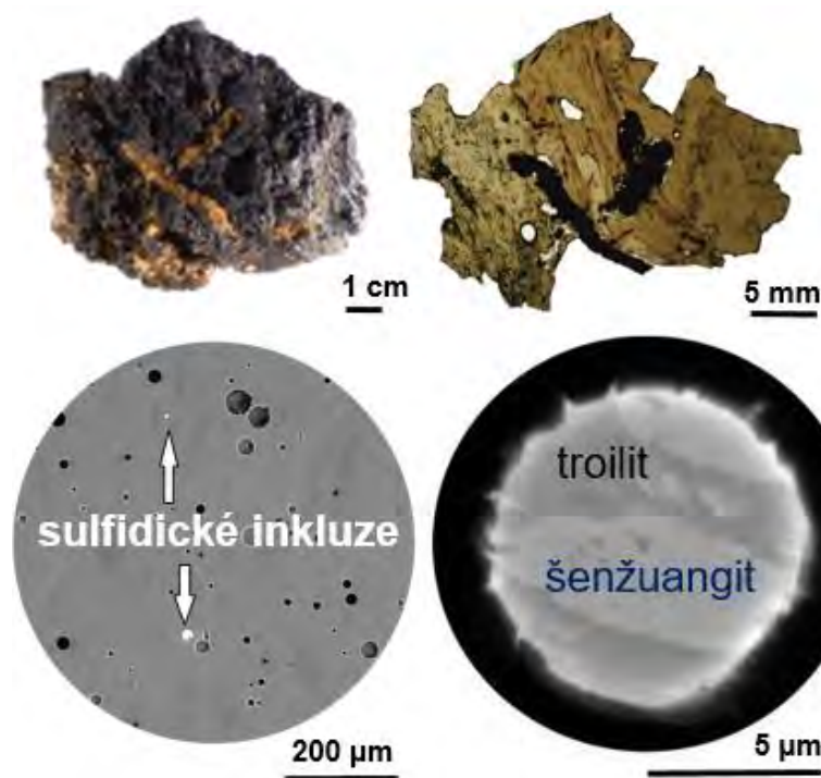
Inkluze v impaktivních sklech (troilit-sulfid železnatý)
