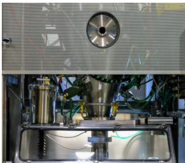
Indukční plazmový systém pro tvorbu nástřiků TEKNA TekSpray 15
